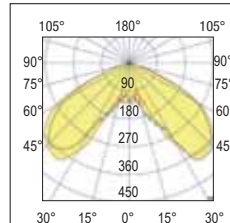
Optica consigliata per illuminazione parchi - Optics recommended for lighting in parks LT-20485
