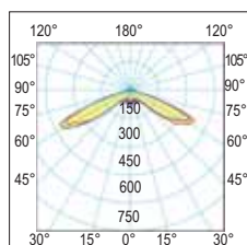
ST/CDL2 Optica consigliata per illuminazione parchi Optics recommended for lighting in parks
