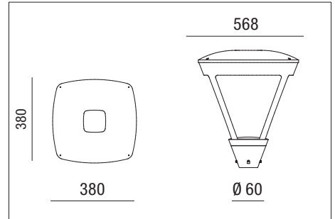
Optica consigliata per illuminazione parchi - Optics recommended for lighting in parks LT-20485
