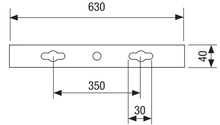
Dimensioni (mm) taffa di fissaggio Mounting bracket dimensions (mm)
