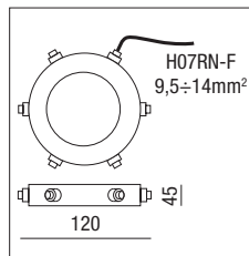
Cod. 12370 Big box - IP68 1 Entrata / 5 Uscite - 1 Input / 5 Outputs
