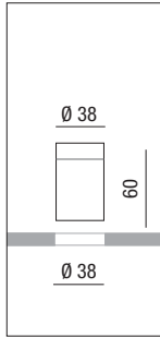
Cod. 27243 Cassaforma per installazioni su muratura. Formwork for walling installations.
