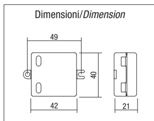
Cod. PTDC/3/350/N 3W
