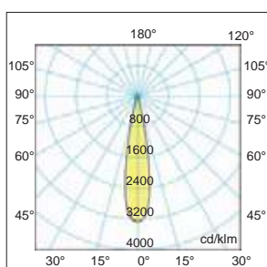
Cod.46011
