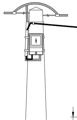
O6CD0 Caixa de distribuição para baixadas T0
