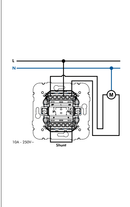
BOTÃO DUPLO DE COMUTAÇÃO DE PERSIANA (Comando de um ponto)
