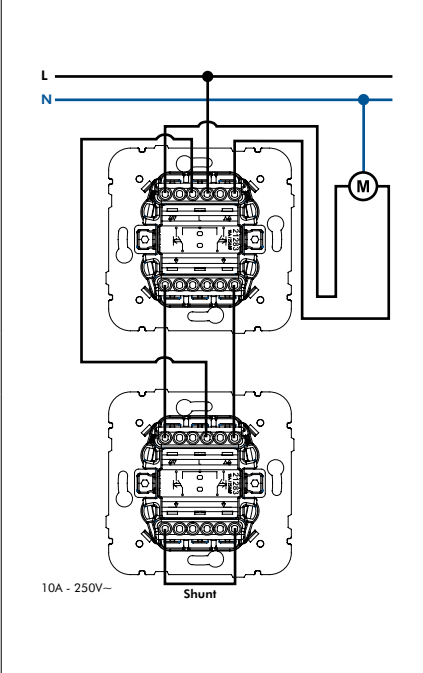
BOTÃO DUPLO DE COMUTAÇÃO DE PERSIANA (Comando de dois ou mais pontos)
