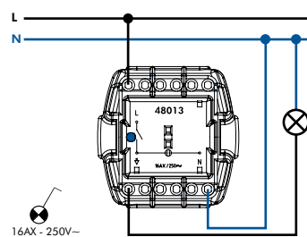
INTERRUPTOR COM SINALIZAÇÃO
