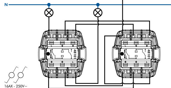
INVERSOR DE GRUPO LUMINOSO
